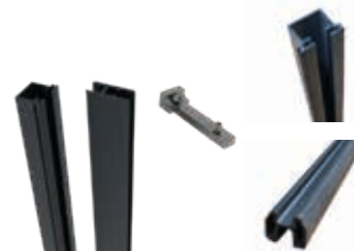
PROFILSET GLAS HORIZONTAL 2 Profile inkl. Konnektoren L175 cm Art.2530
