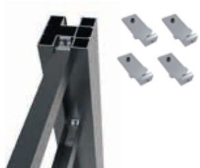
START/ENDPROFIL (lose) 25 x 30 x 1750 mm benötigt werden 2 St. je Zaunfeld ANTHRAZIT - Art.2644 SCHWARZ - Art.2828
